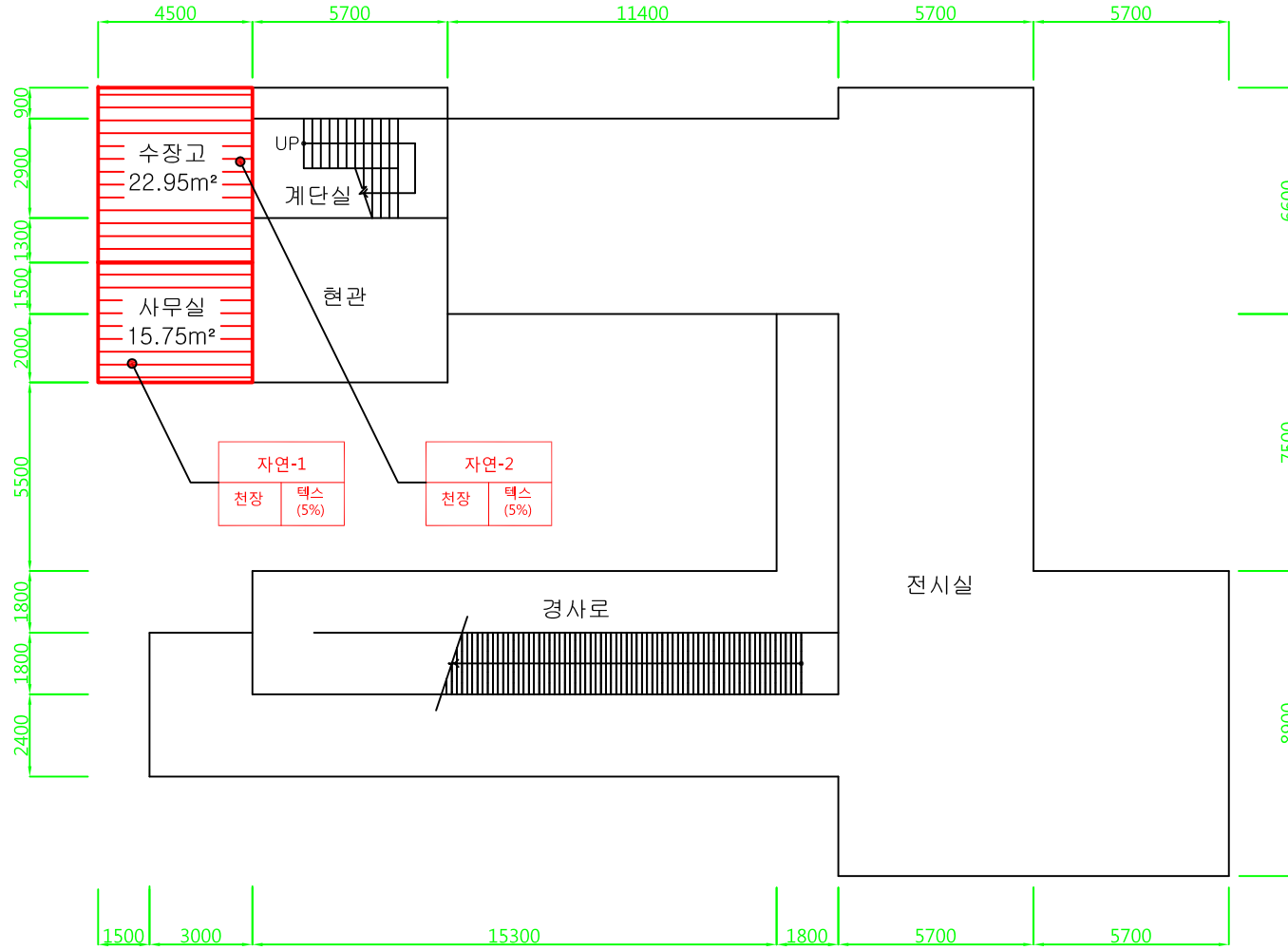
○ 당항포자연사박물관 지상1층평면도
