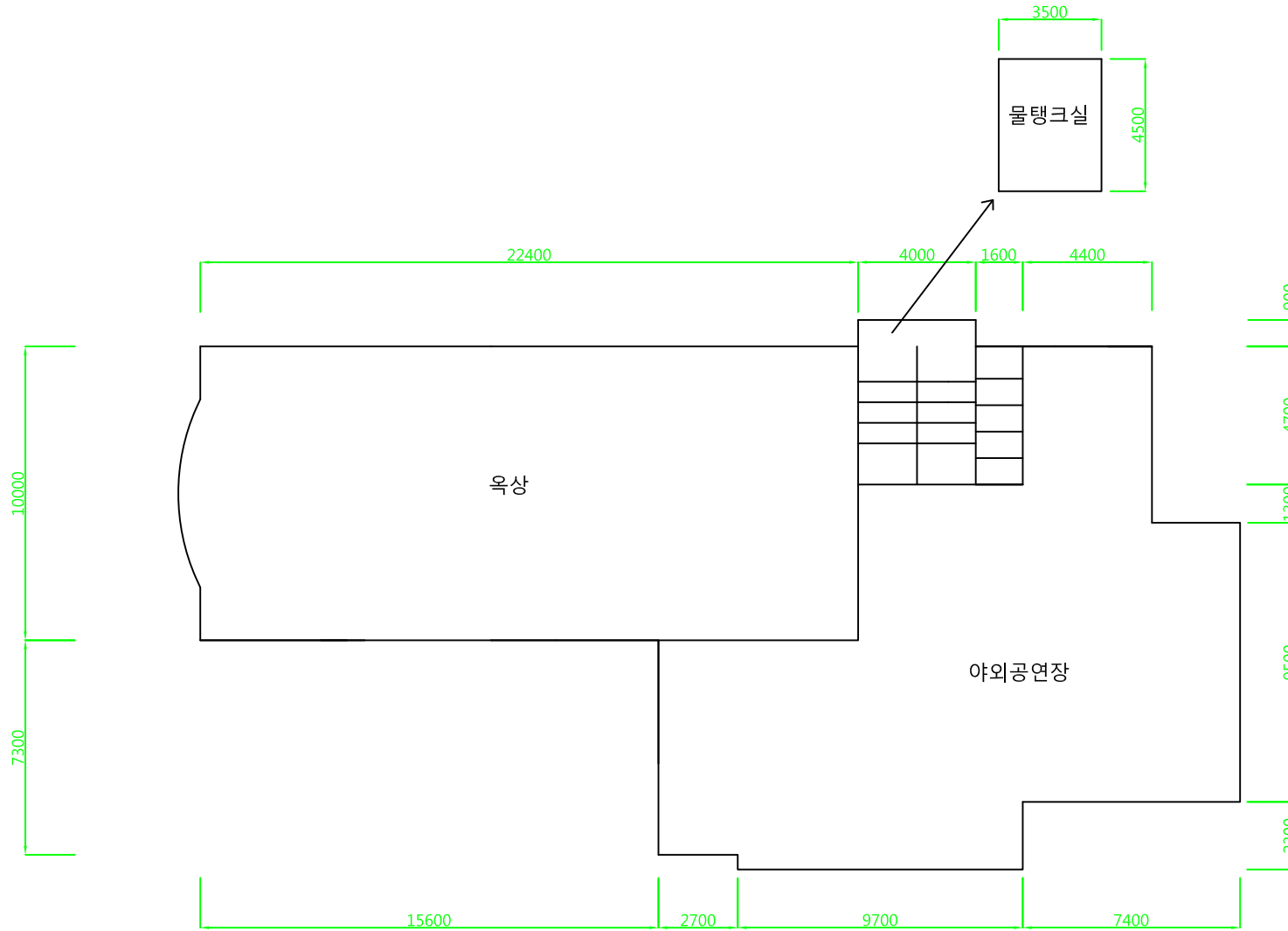
고성동부도서관 옥상 평면도
