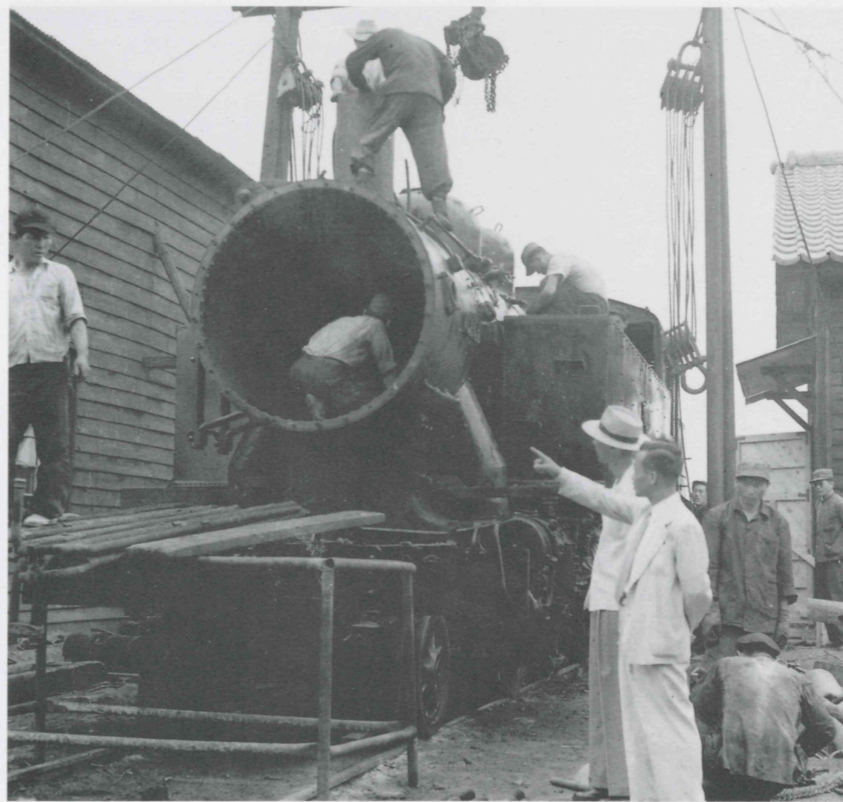
우리나라 최초로 열차조립을 마치고 시운전에 앞서 화이팅을 외치고 있는 제작진들.(53. 7. 20) 우리나라 기술진이 열차를 조립하고 있다.(53. 7. 20)
